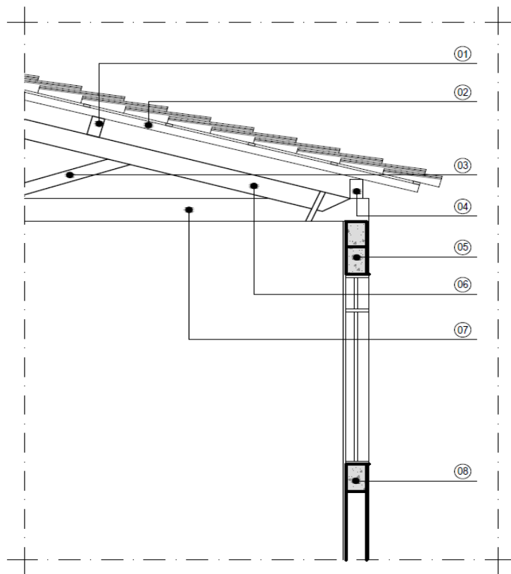
1 CORTE ESQUEMÁTICO DE COBERTURA E JANELA SEM ESCALA
