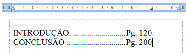
FIGURA 1 – Parágrafo formatado
