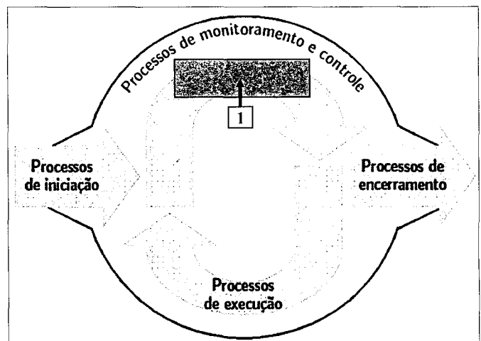
Figura 3 - Processos PMBOK
