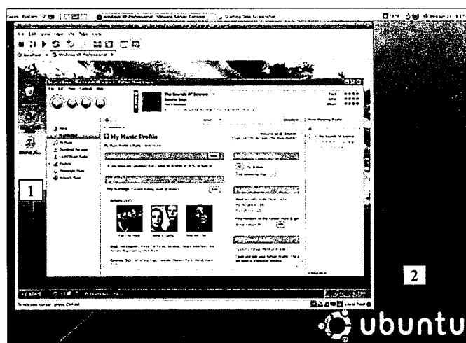
Figura 11 - Windows XP
