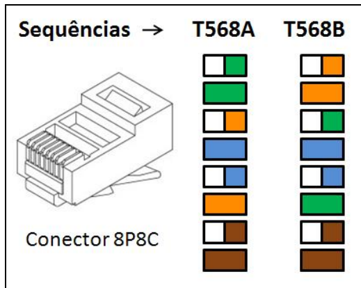
Figura 1 – Duas sequências de cores de fios para conectores 8P8C, de acordo com o padrão EIA/TIA-568-B.
